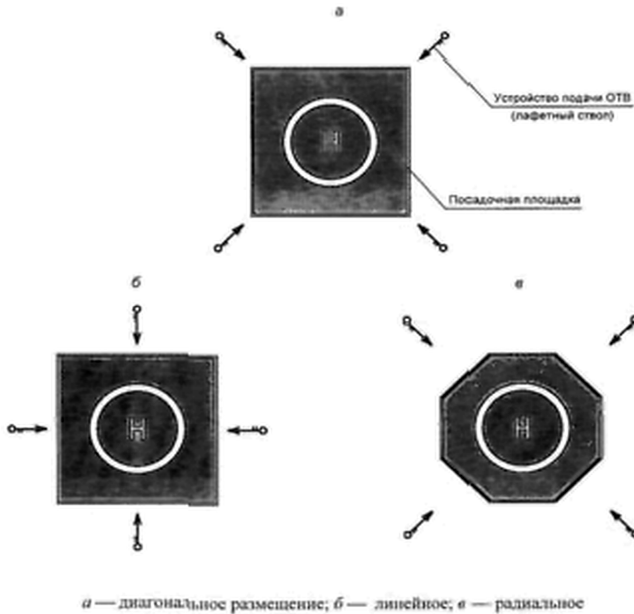
"Рис. А.1. Схемы размещения стационарных лафетных стволов"
