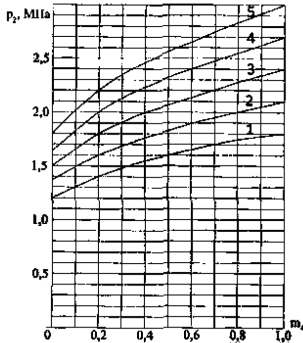
Рисунок Б.1. Зависимость давления p_2 в изотермическом резервуаре в конце выпуска расчетного количества двуокиси углерода m от относительной массы двуокиси углерода m_4
